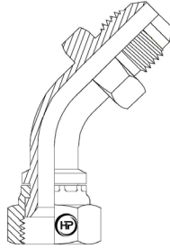
JICM X JICF 45° BEND (M X F)
