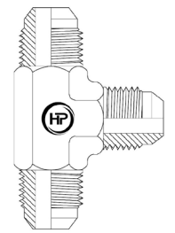
JICM X JICM X JICM EQUAL TEE
