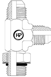
JICM X UNOM X JICM RUN TEE
